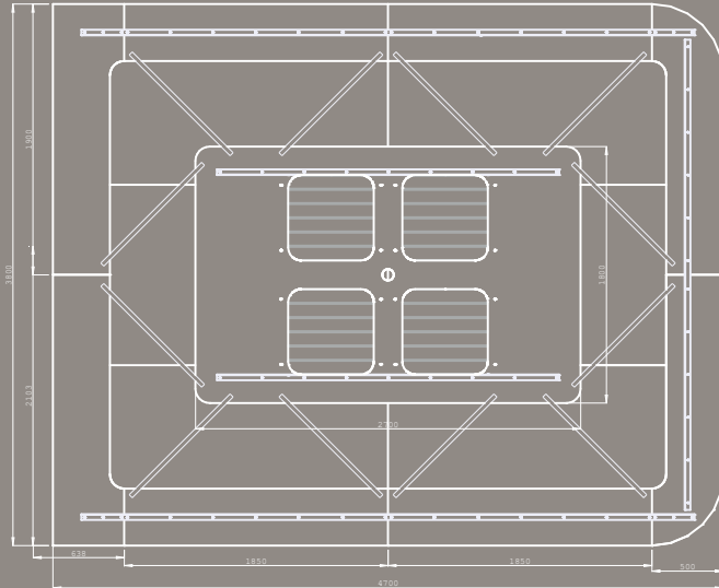
Púdorys - spodni časť
